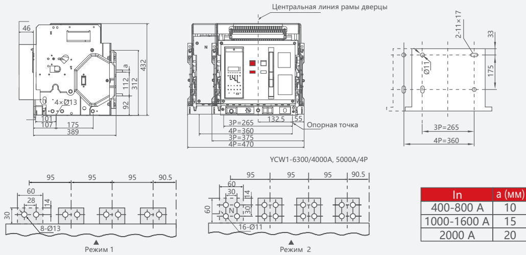
Габаритные размеры автоматического выключателя выкатного типа YCW1-2000A
