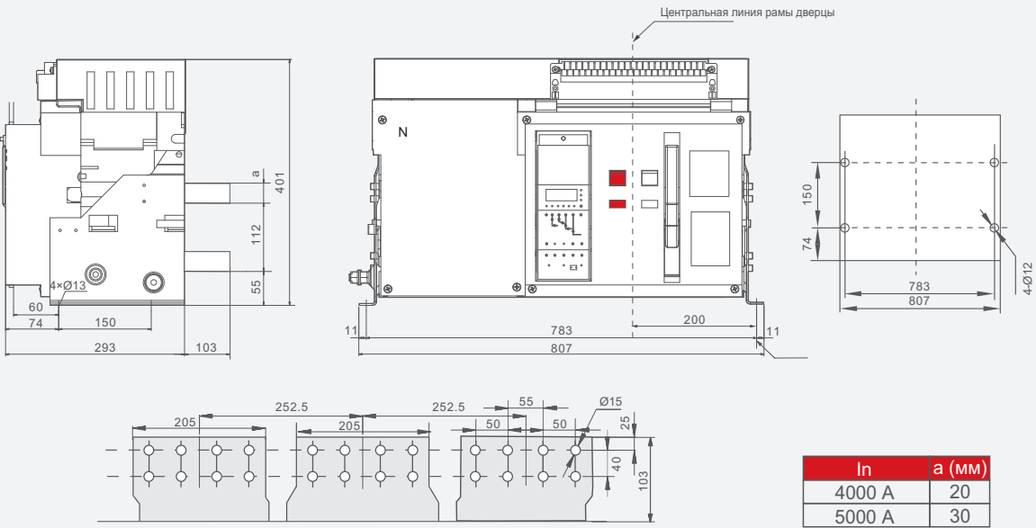
Габаритные размеры YCW1-6300/3P
