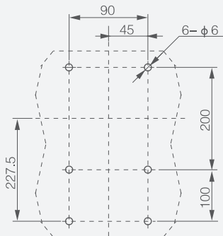
4P: монтаж на панель
