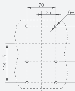
4P: монтаж на панель
