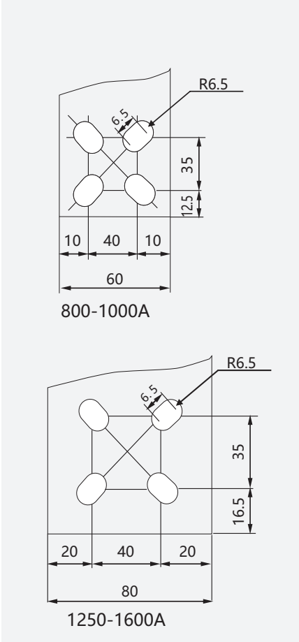
Схема монтажа 1000-1600 А
