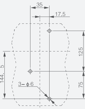
3P: монтаж на панель
