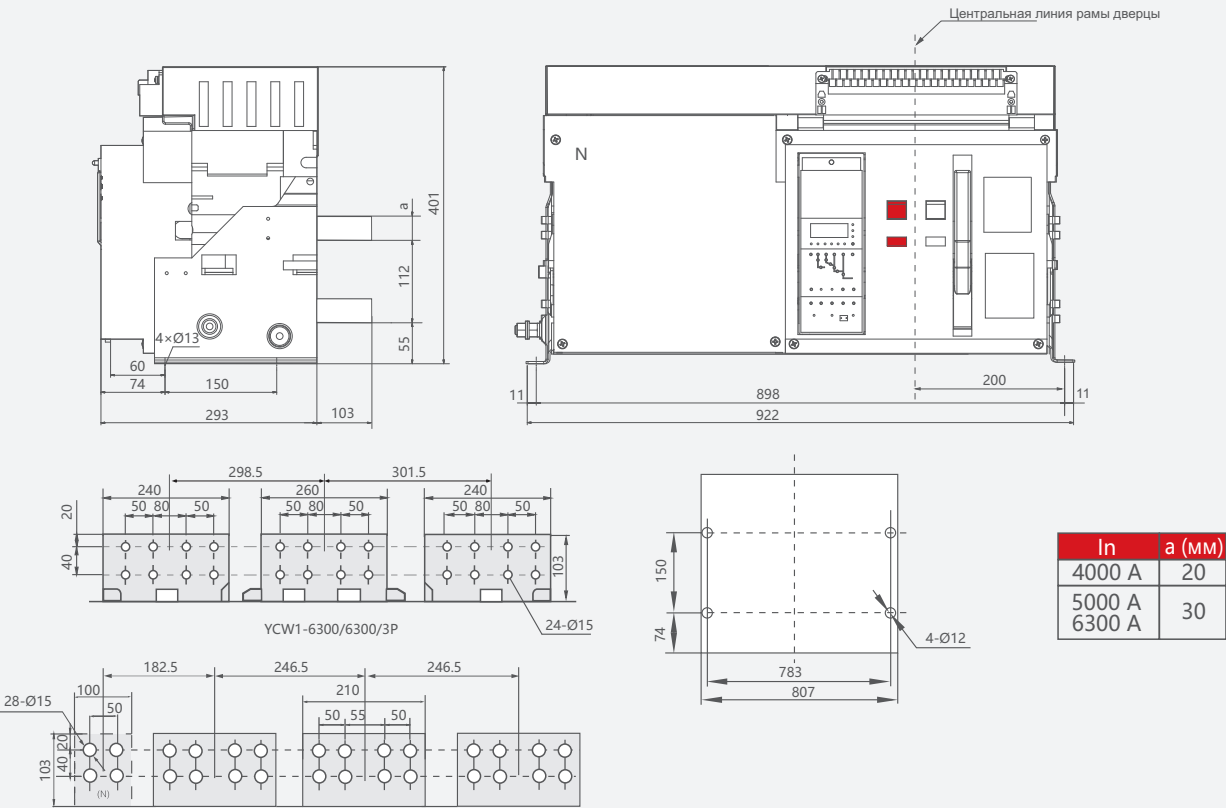
Габаритные размеры стационарного выключателя YCW1-6300A
