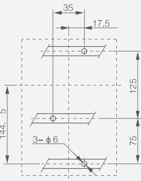
3P: монтаж на направляющие
