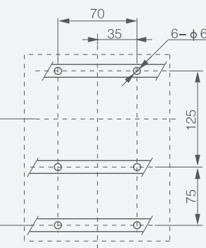
4P: монтаж на направляющие
